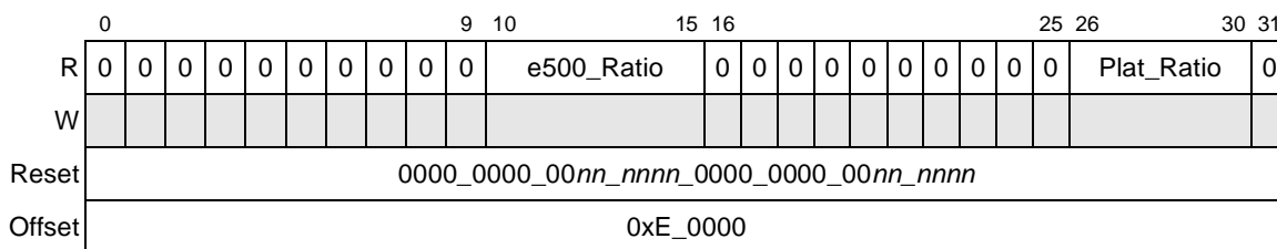
Figure 18-1. POR PLL Status Register (PORPLLSR)
